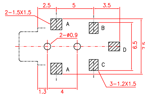
印制板开孔示意图
