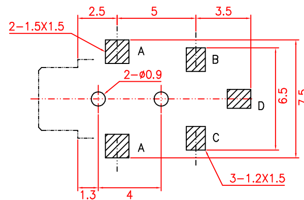
印制板开孔示意图
